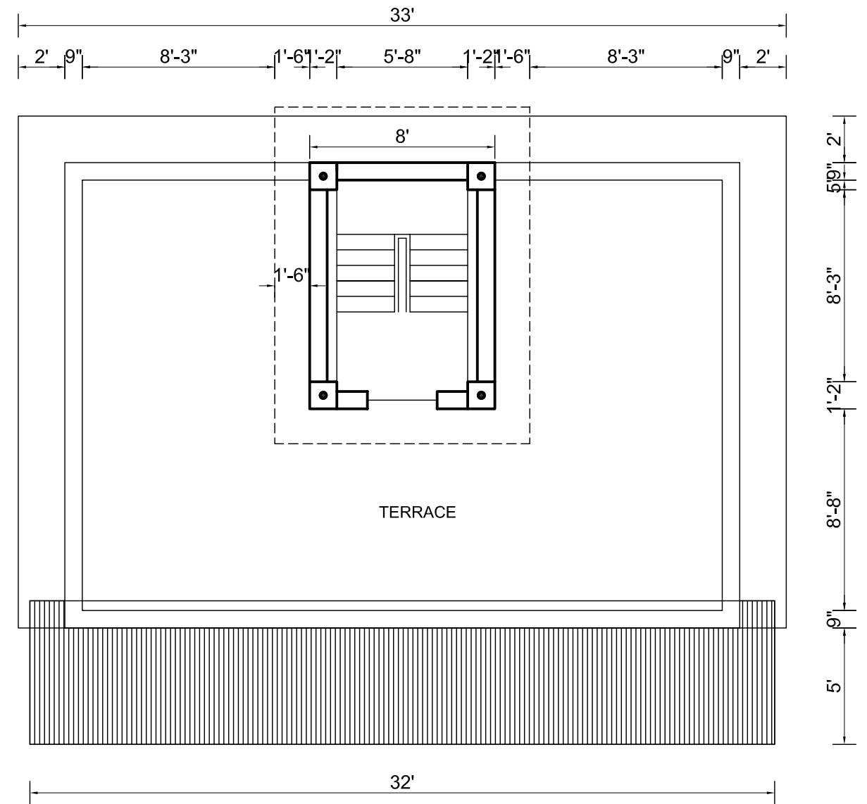
TOPFLOOR PLAN
